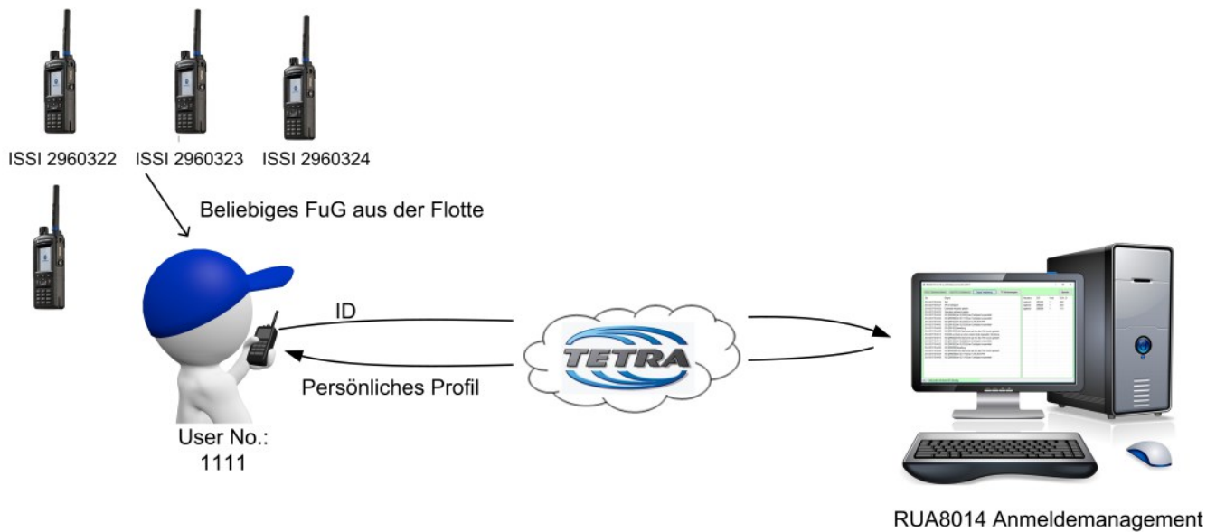
Abb. Systemübersicht RUA8014
